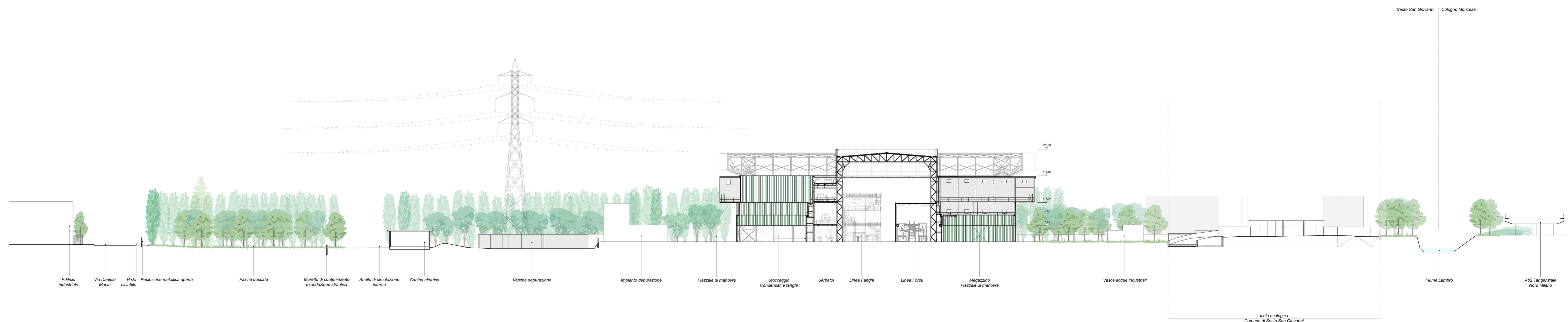
PROGETTO - SEZIONI GENERALI 4 - 4
