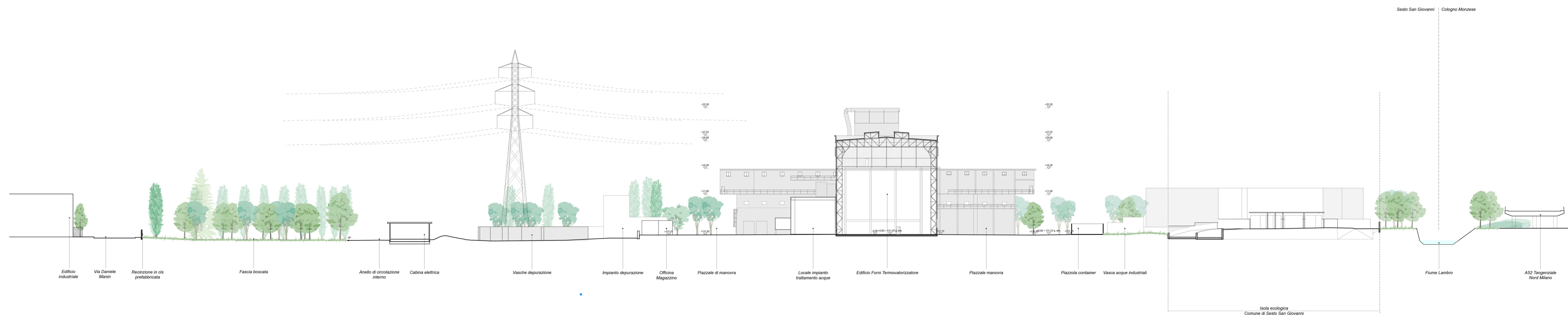
STATO DI FATTO - SEZIONI GENERALI 4 - 4
